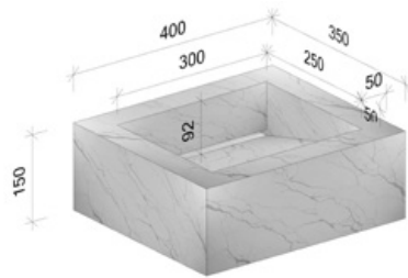
WT wandhängend (unterbaufähig) Integrated top with 1 washbasin (under buildable)
