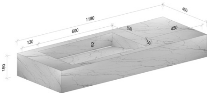
WT wandhängend (unterbaufähig) Integrated top with 1 washbasin (under buildable)
