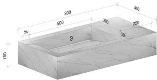
WT wandhängend (unterbaufähig) Integrated top with 1 washbasin (under buildable)
